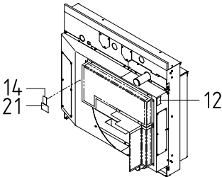
FAN SHROUD
